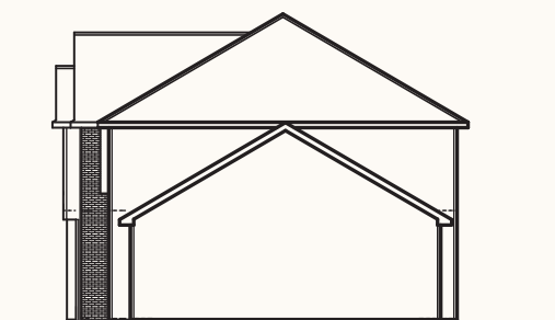
RIGHT ELEVATION
